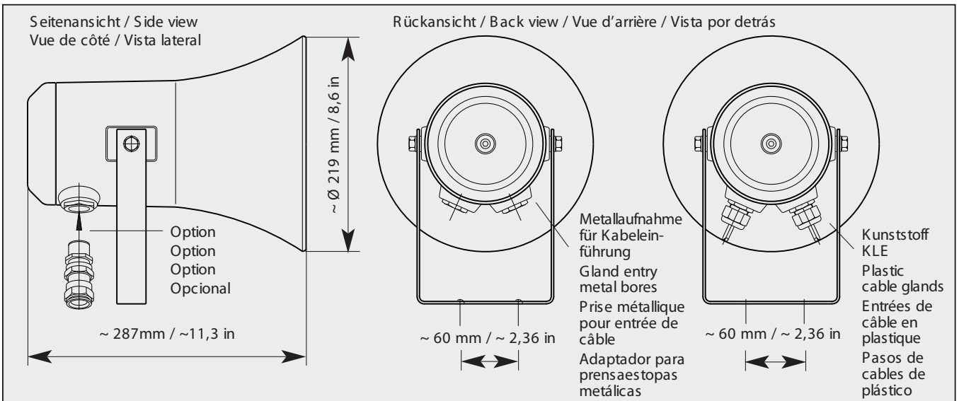
Maßbild / Dimensions / Dimensions / Hoja de cotas
